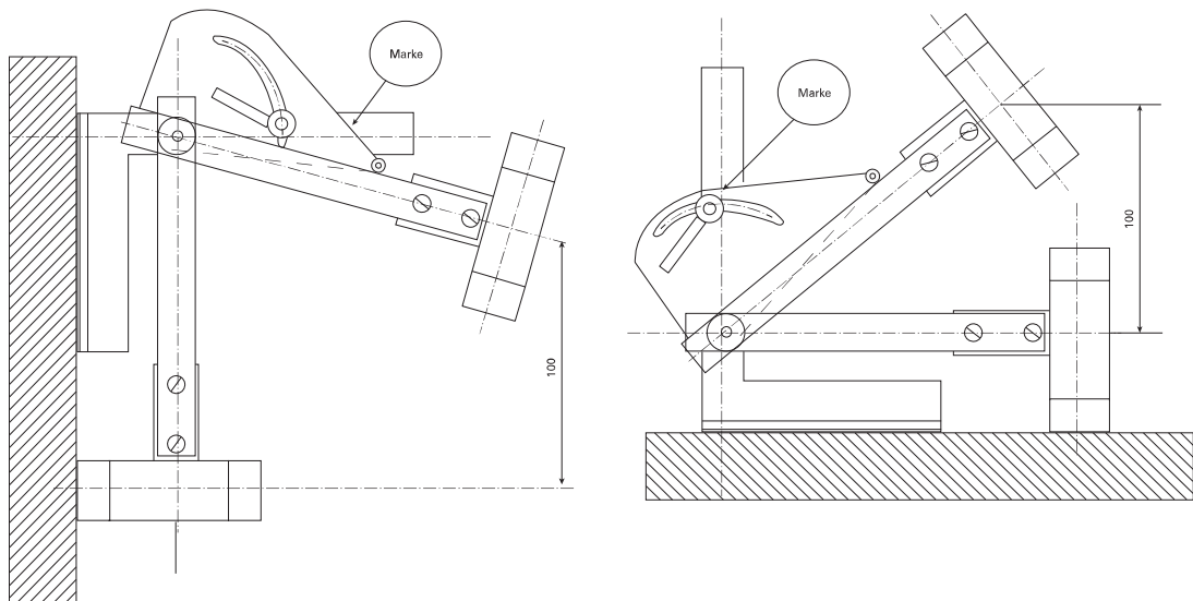
Fallhammer an senkrechter Fläche (Horizontalschlag)
