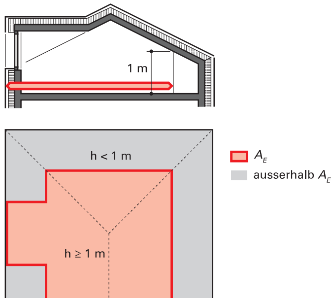
Figur 8 Energiebezugsfläche in Dachgeschossen
