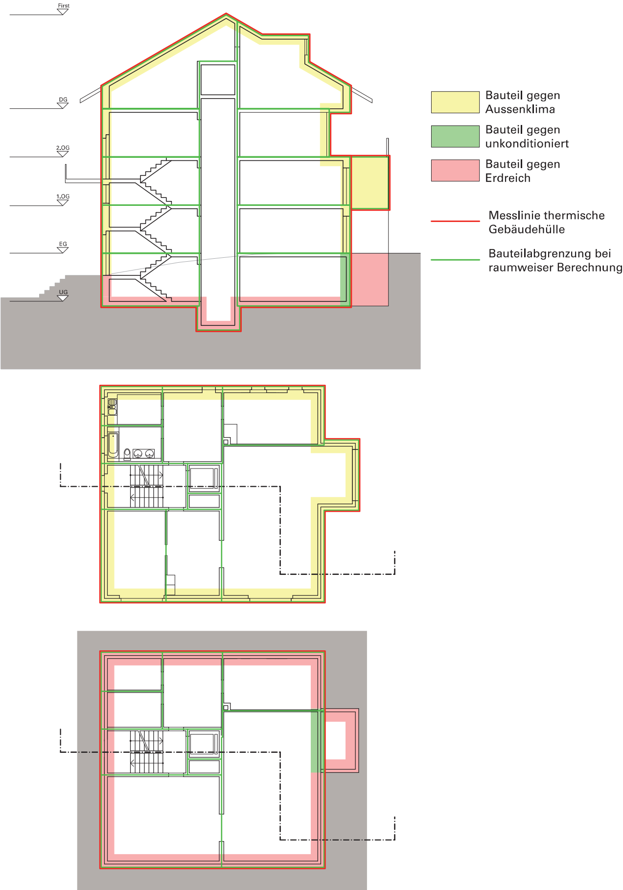
Figur 4 Beispiel eines Schnitts und je eines Grundrisses 1. OG und UG
