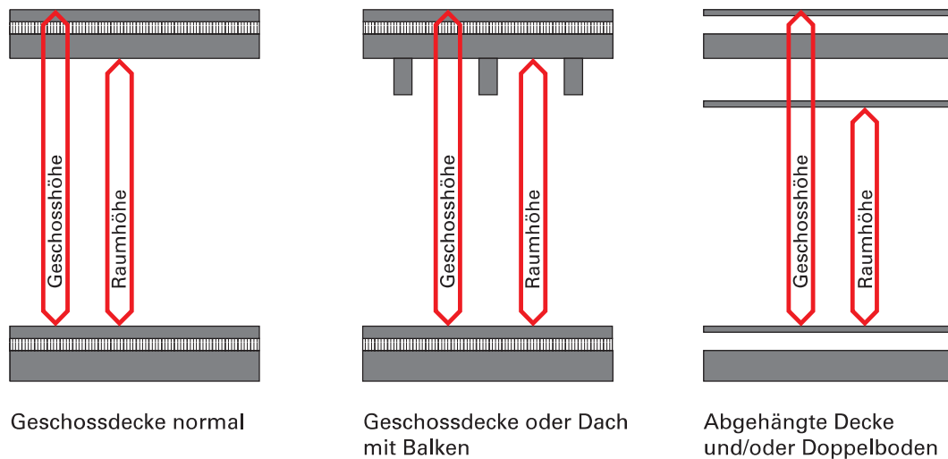
Figur 2 Geschosshöhe und Raumhöhe
