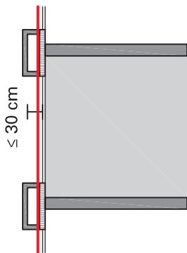
Figur 6 Messebene der thermischen Gebäudehülle bei Gebäudevorsprüngen und Balkonen (Grundrisse)
