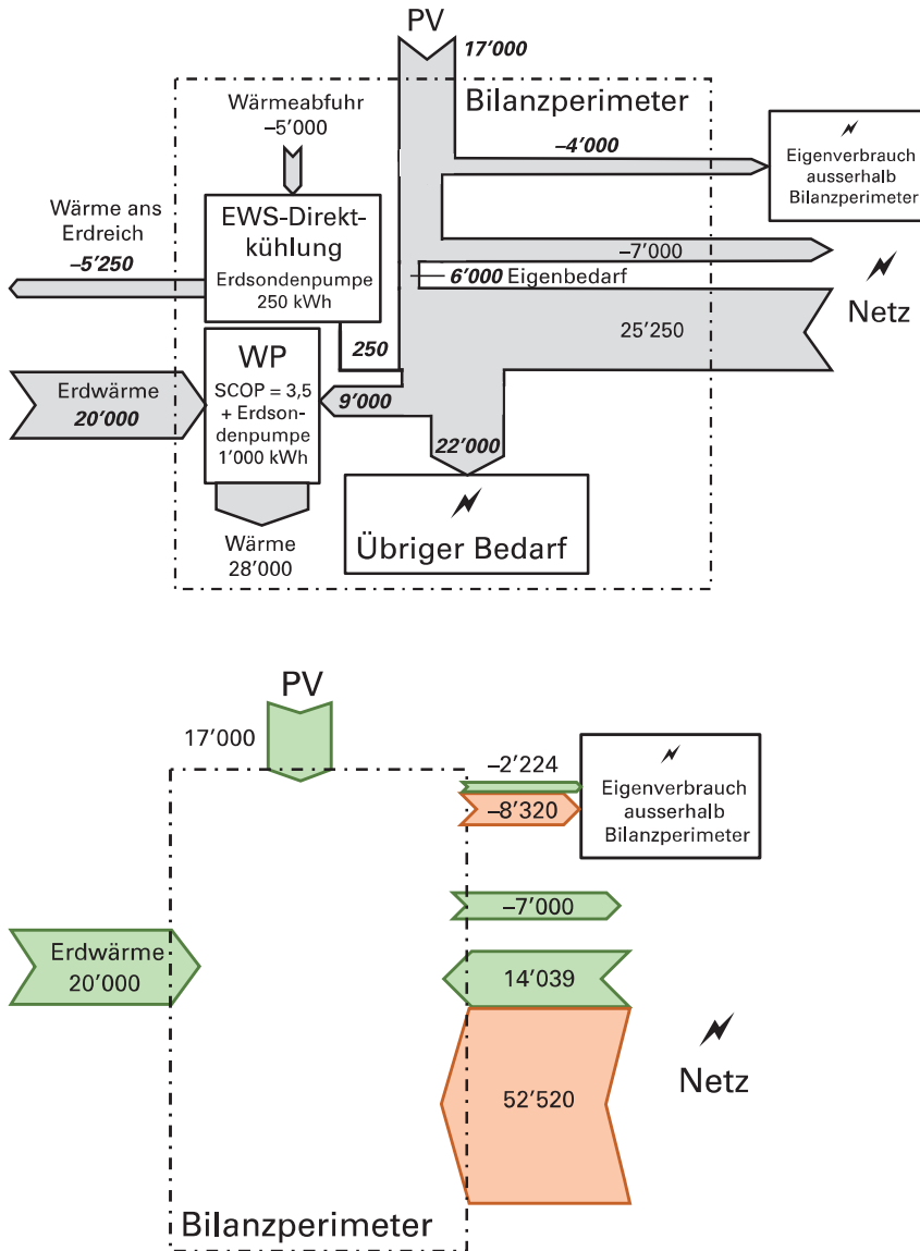
Figur 10 Energieflüsse zu Beispiel 2 in Tabelle 9 (alle Werte in kWh); oben: physikalische Flüsse (fett und kursiv gedruckte Werte sind Eingabewerte); unten: bilanzierte, bewertete Flüsse (Primärenergie, grün: erneuerbar, rot: nicht erneuerbar)
