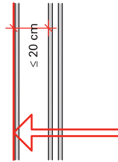
Figur 5 Messebene der thermischen Gebäudehülle (Schnitte) (Fortsetzung)
