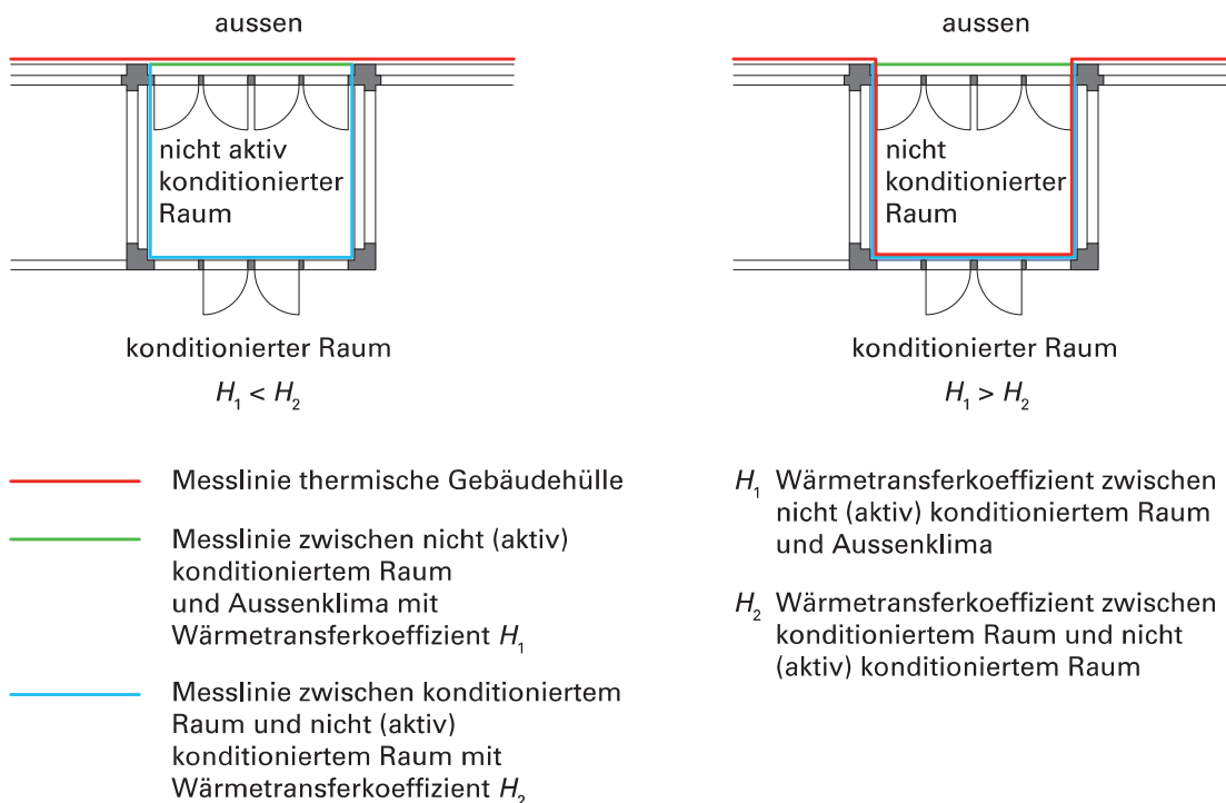
Figur 3 Lage der thermischen Gebäudehülle bei nicht konditionierten Räumen
