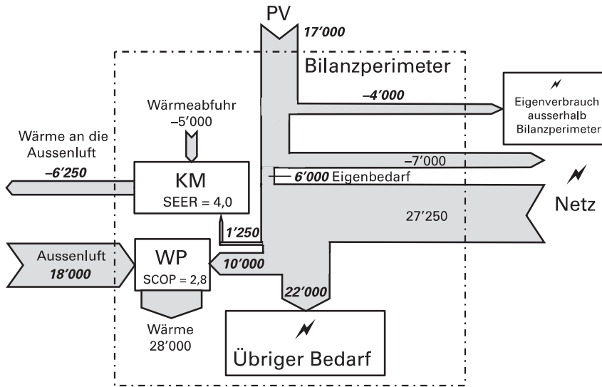
Figur 11 Energieflüsse zu Beispiel 3 in Tabelle 10 (alle Werte in kWh); oben: physikalische Flüsse (fett und kursiv gedruckte Werte sind Eingabewerte); unten: bilanzierte, bewertete Flüsse (Primärenergie, grün: erneuerbar, rot: nicht erneuerbar)
