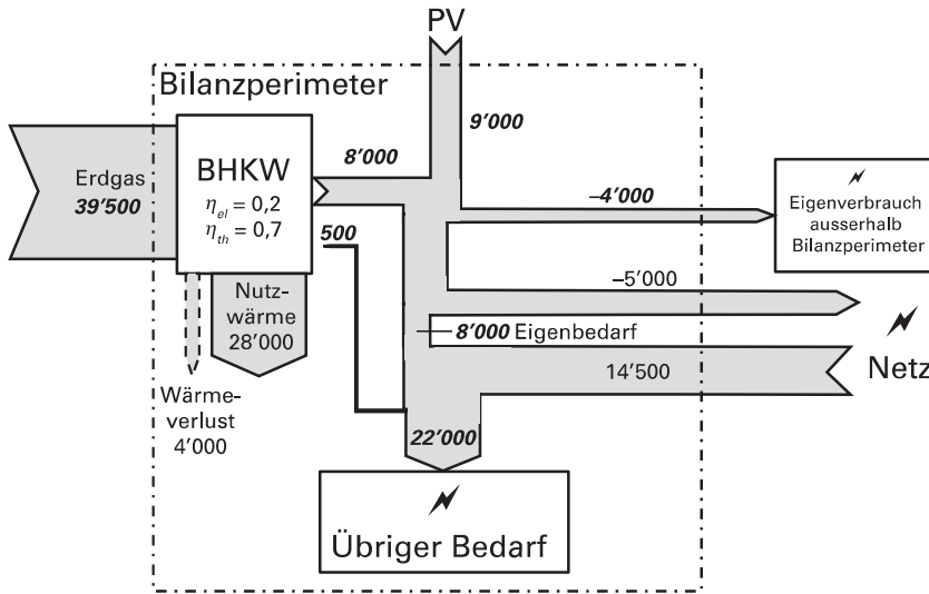
Figur 9 Energieflüsse zu Beispiel 1 in Tabelle 8 (alle Werte in kWh); oben: physikalische Flüsse (fett und kursiv gedruckte Werte sind Eingabewerte); unten: bilanzierte, bewertete Flüsse (Primärenergie, grün: erneuerbar, rot: nicht erneuerbar)
