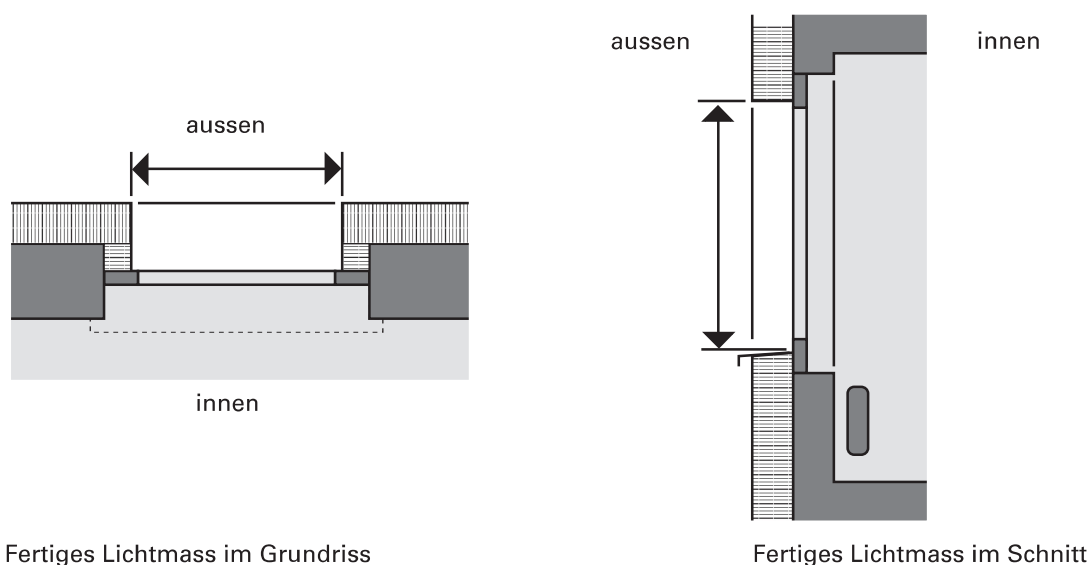
Figur 1 Fenstermass (Grundriss und Schnitt)
