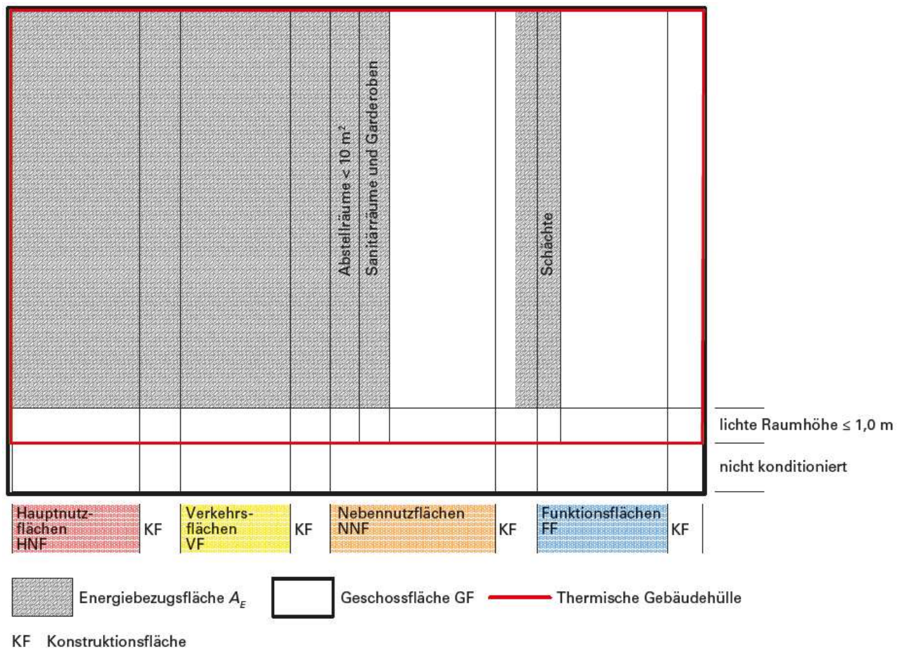
Figur 7 Schema der zur Energiebezugsfläche gehörenden Geschossflächen
