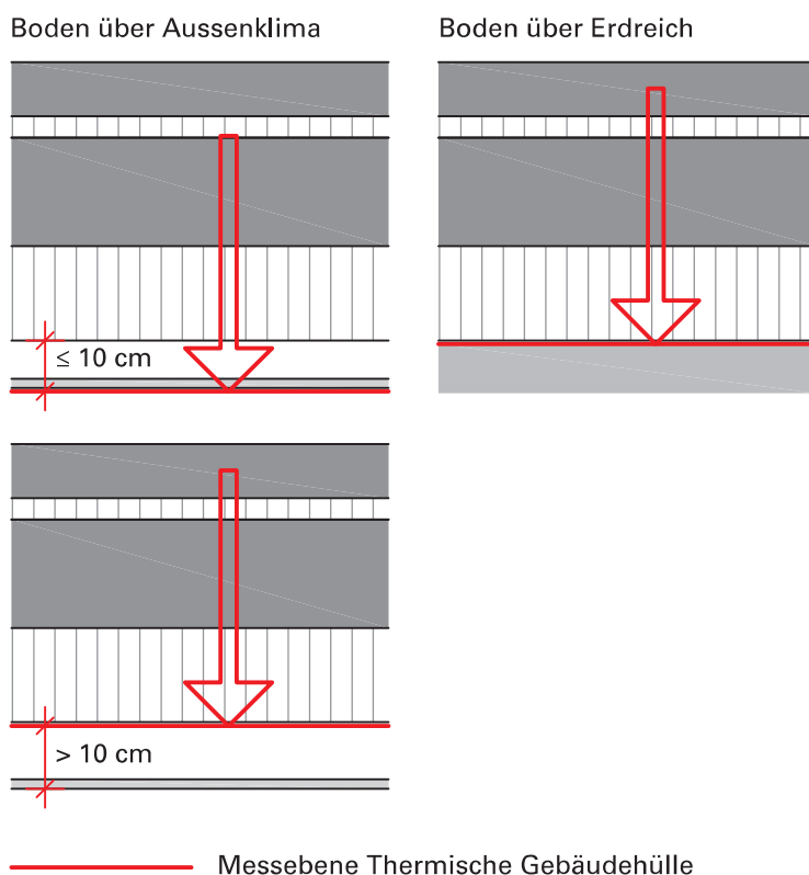
Figur 5 Messebene der thermischen Gebäudehülle (Schnitte)
